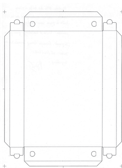
Vue en mode plan de la boîte à pizza sans illustration.
