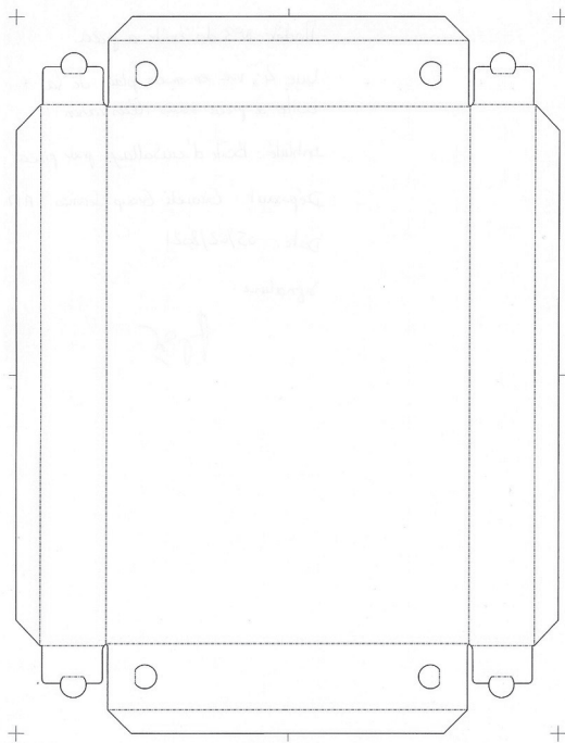
Vue en mode plan de la boîte à pizza sans illustration.
